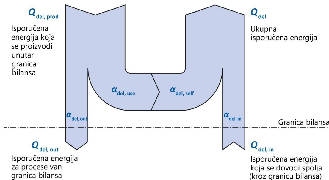
Slika 6 – Bilans isporučene energije
