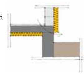
Slika 17: Moguća pojava toplotnog mosta na dijelu sokle
