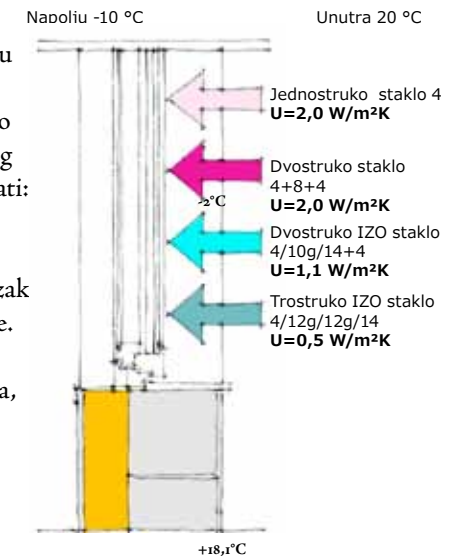
Slika 26: Temperature na unutarnoj površini stakla u zavisnosti od vrste ostakljenja / Izvor: "Priručnik za energetske savjetnike"-Program Ujedinjenih naroda za razvoj (UNDP) u Hrvatskoj /
