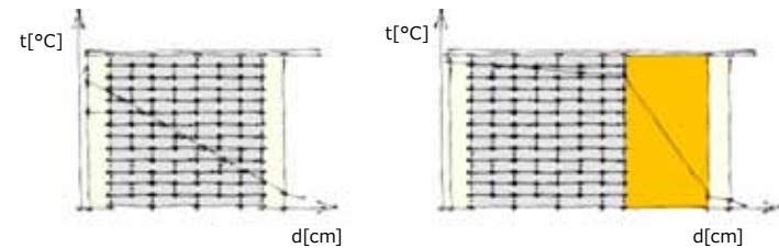
Slika 15: Krive izolovanog i neizolovanog betonskog zida
