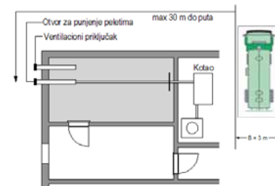
Slika 31: Osnova prostora za smještaj peleta i mogućnost prilaza cistijerni
