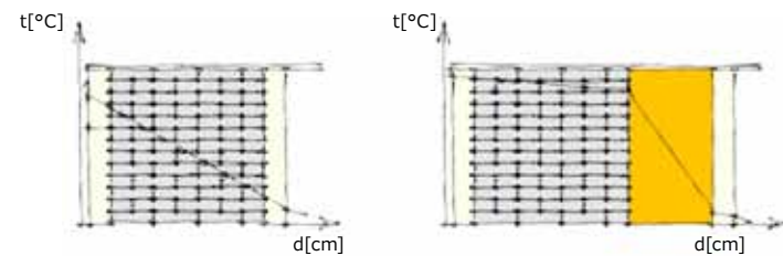
Slika 14: Krive izolovanog i neizolovanog zida od opeke
