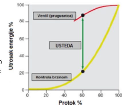
Slika 41: Ušteda energije upotrebom frekventne regulacije
