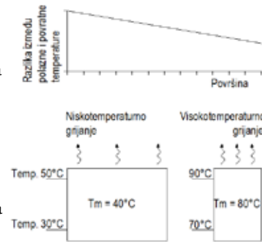
Slika 30: Zavisnost površine grejnih tijela od temperature vode u razvodnom sistemu
