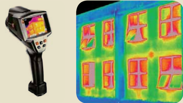
Slika 7: Termografska kamera i rezultat mjerenja (termogram)
